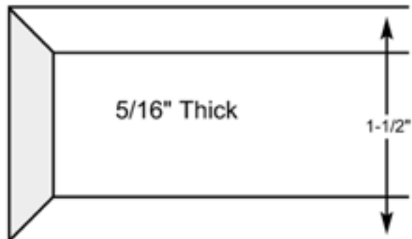
Double Bevel
